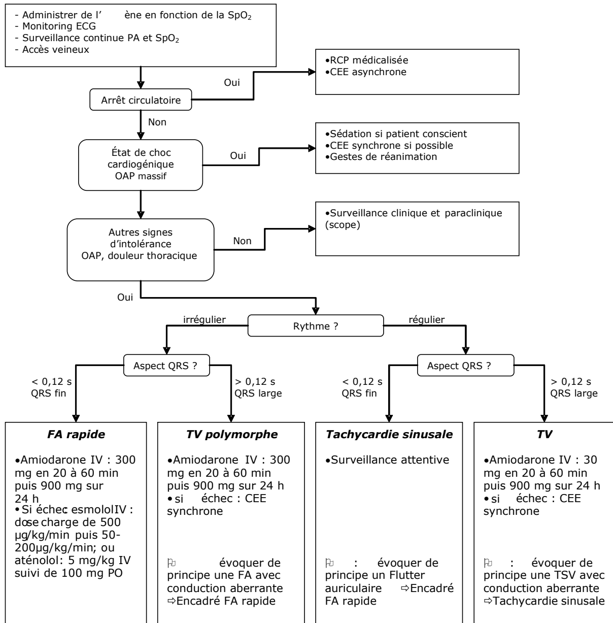
Algorithme 4. Algorithme thérapeutique de la tachycardie (fréquence cardiaque > 100 bpm) chez un patient présentant un SCA, hors défaillance vitale et tachycardie bien tolérée (d'après JE de la Coussaye et al. cf. texte d'expert).
